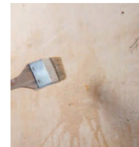
Benetzungsprobe Prüfen der Saugfähigkeit des Untergrundes
